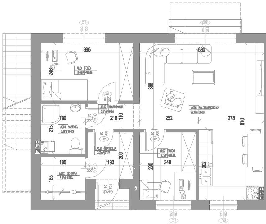
RZUT PARTERU LOKAL A
