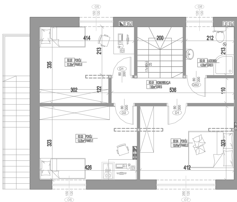
RZUT PODDASZA LOKAL B
